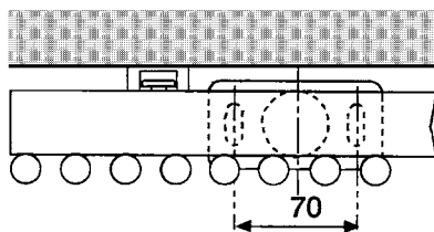
KLVD (vista dall'alto)
