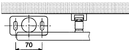
KLH (vista dall'alto)
