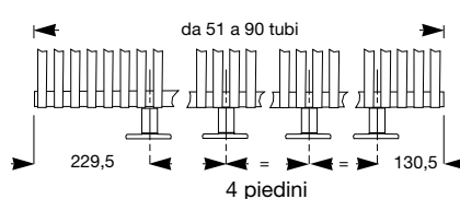
Piedino KLV/KLVD
