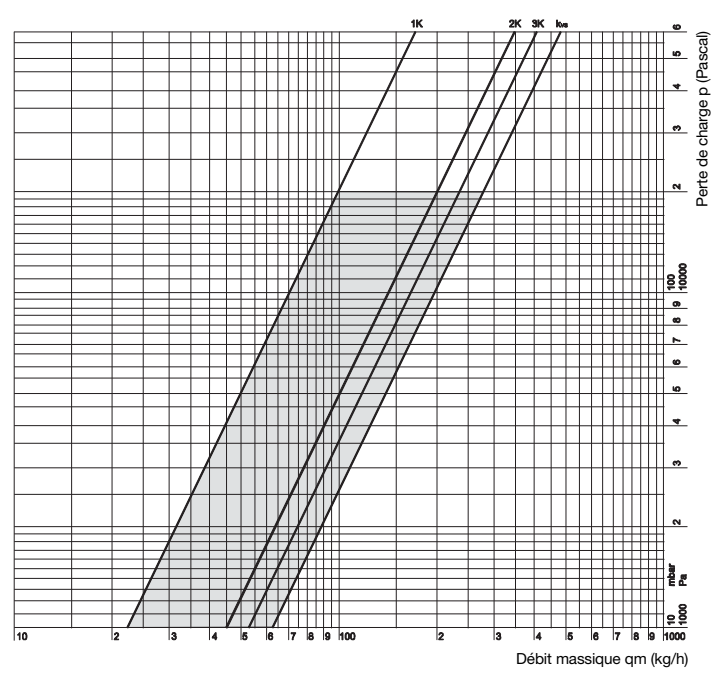
Diagramme de perte de charge du thermostat de forme axiale (Honeywell MNG)
