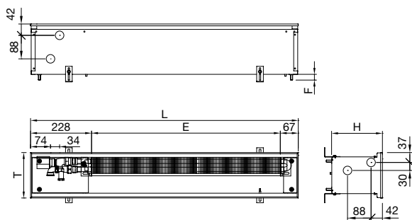
Figure sans grille, cotes en mm Vannes et actionneur non fournis à la livraison
