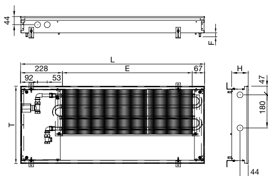
Figure sans grille, cotes en mm Vannes et actionneur non fournis à la livraison
