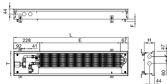
Figure sans grille, cotes en mm Vannes et actionneur non fournis à la livraison
