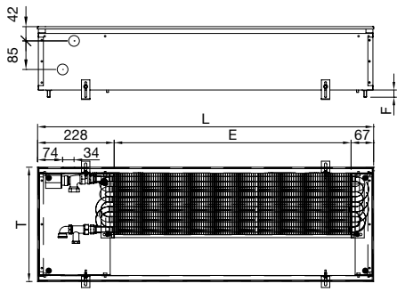
Figure sans grille, cotes en mm Vannes et actionneur non fournis à la livraison
