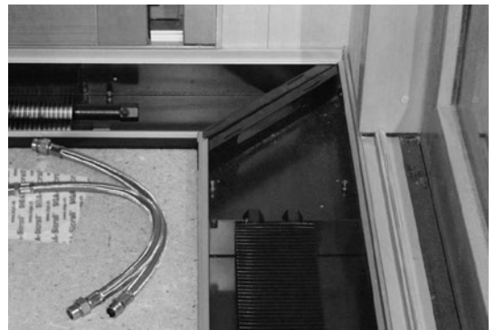
Exemple de couplage avec tuyau flexible, selon un angle de 90°, éventuellement possible sur demande et selon le modèle
