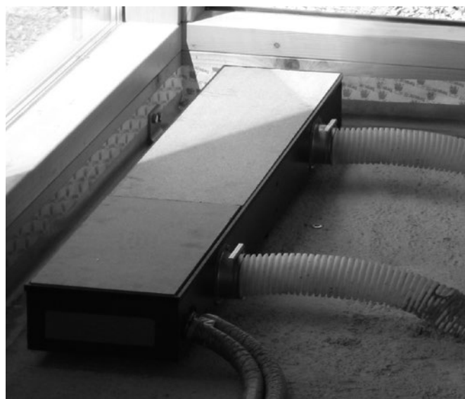
Position du raccordement d'air frais
