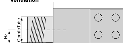
Détail de raccordement du conduit de ventilation
