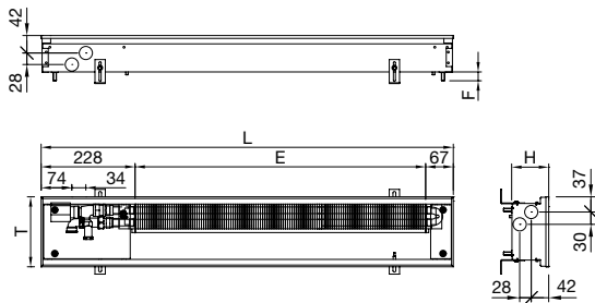
Figure sans grille, cotes en mm Vannes et actionneur non fournis à la livraison
