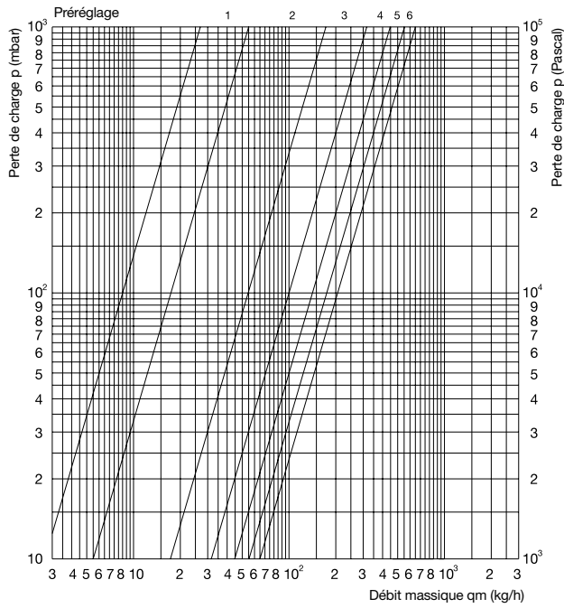
Diagramme de perte de charge de l'insert de vanne AV6 (Oventrop)
